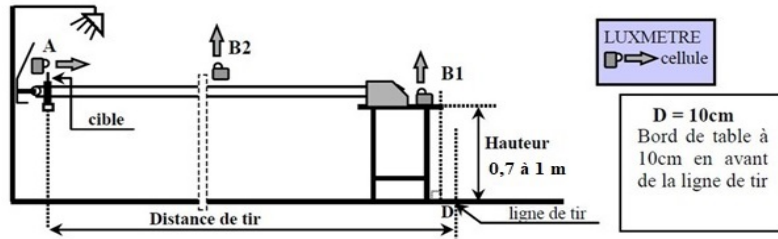
Mesure de l'éclairage des stands intérieurs
