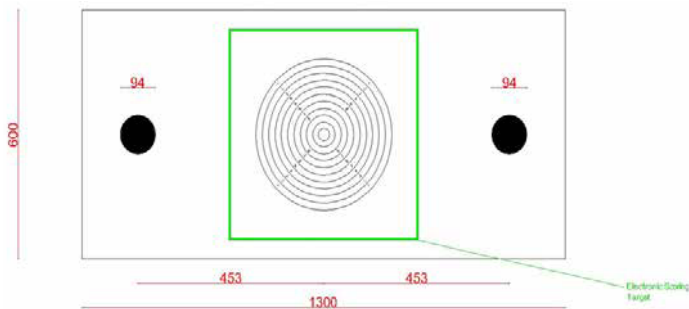
Cible pour Cible Mobile 50m avec EST
