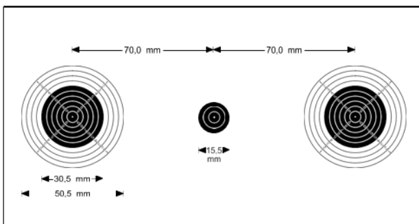
Cible papier pour Cible Mobile 10m
