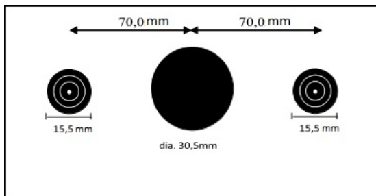
Cible pour Cible Mobile 10m avec EST
